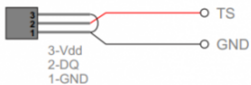
DS18B20 wiring diagram
