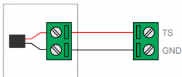
DS18B20 wiring diagram
